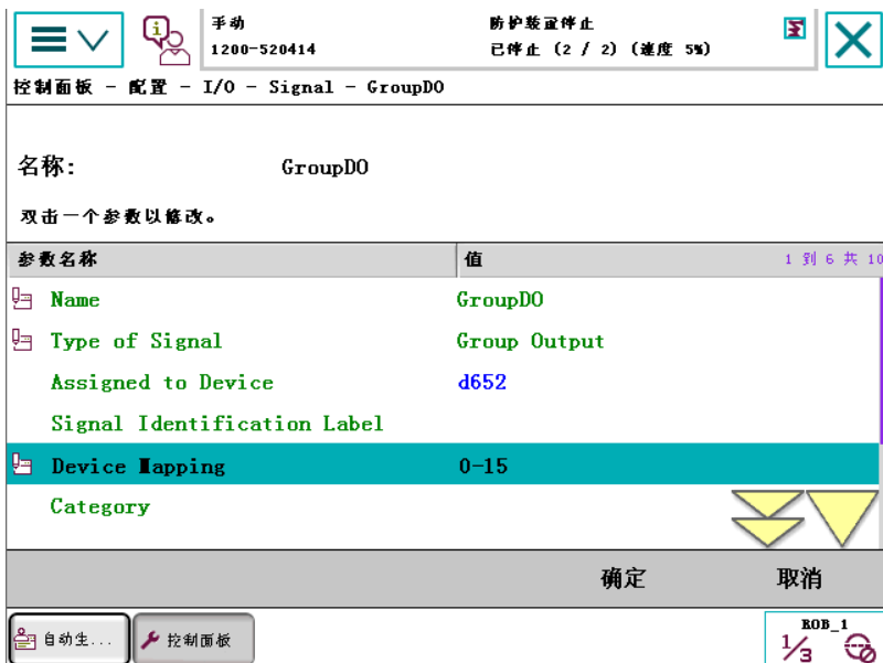
图 18: 示教器添加 GroupDO 端口
