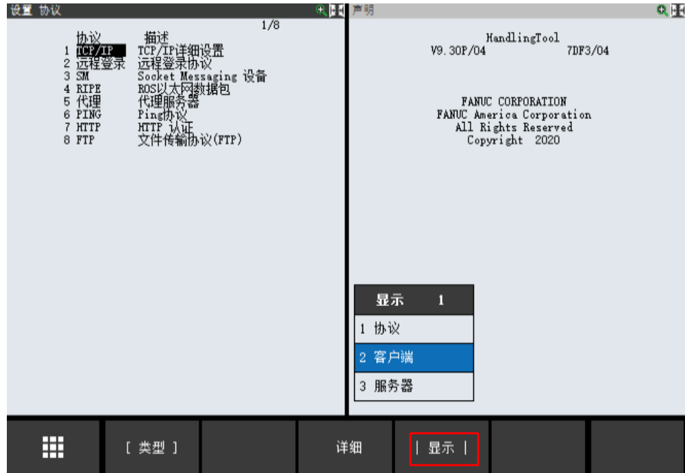
图 46: fanuc 设定机械臂机械臂主控 socket 1
