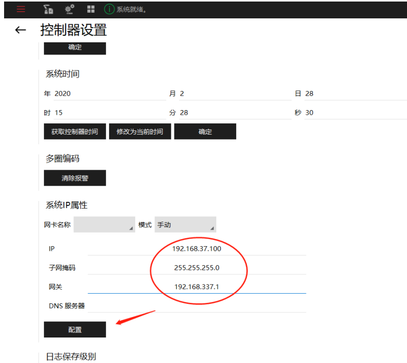
图 86: ROKAE 设定机械臂 IP
